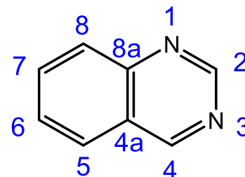
Chinazolin (quinazoline)
