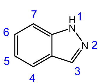
1H-Indazol
