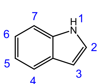
1H-Indol
