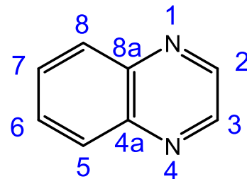
Chinoxalin (quinoxaline)
