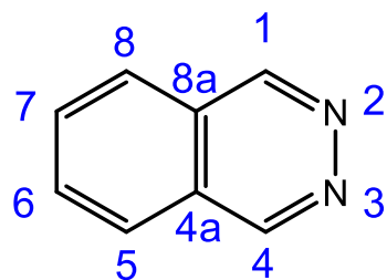
Phthalazin
